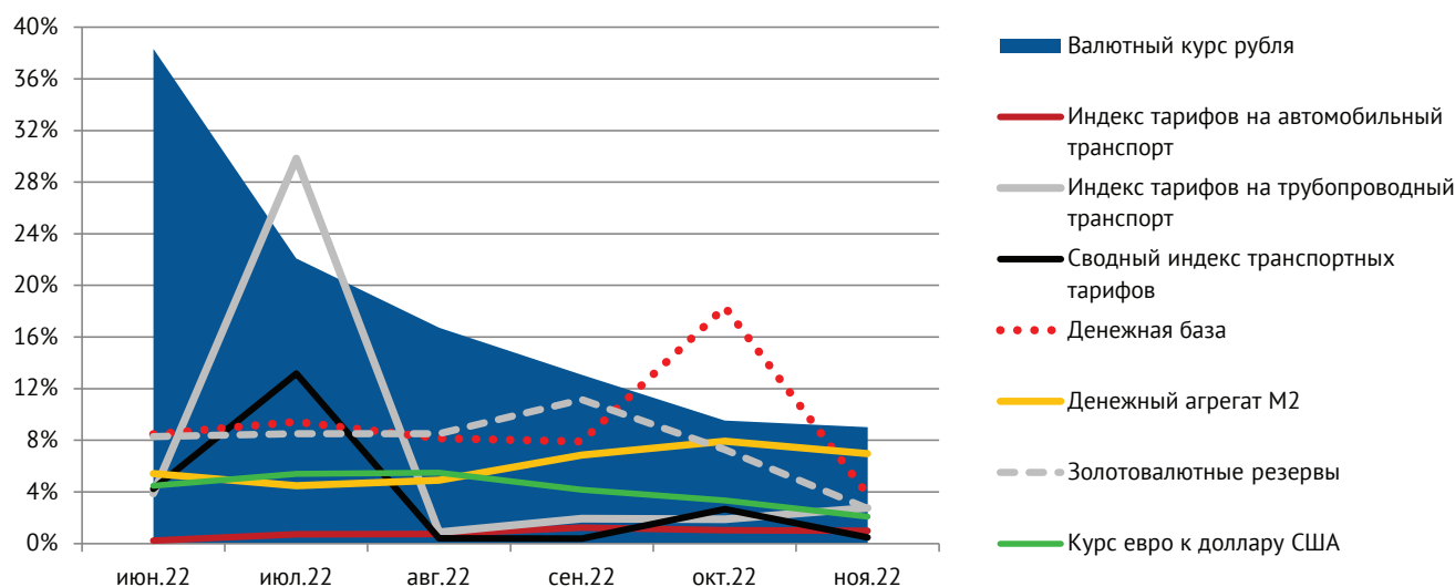
Рис. 1. Средняя абсолютная процентная ошибка прогнозов в июне-ноябре 2022 г.
