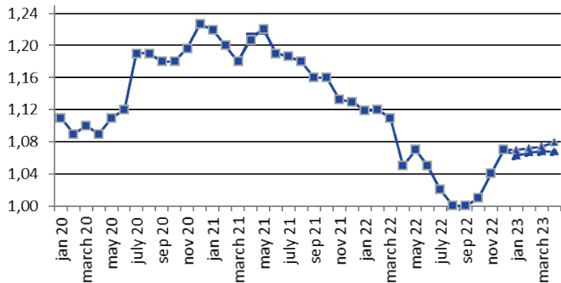
Рис. 41. Курс USD/EUR
